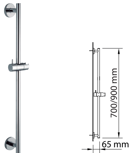
STYLE BARRA DE DUCHA Sliding bar Barre de douche
