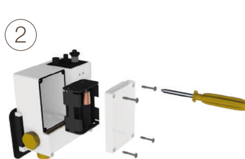
Cambio de pilas Change the batteries / Changement de piles
