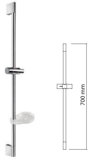
MALAWI ø20x700 mm BARRA DE DUCHA Sliding bar / Barre de douche
