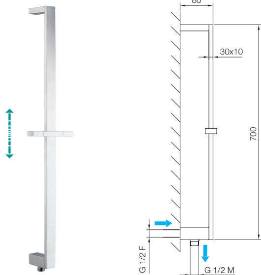
TREND - 30x10x700 mm BARRA DE DUCHA EMPOTRADA Concealed sliding bar Barre de douche encastré
