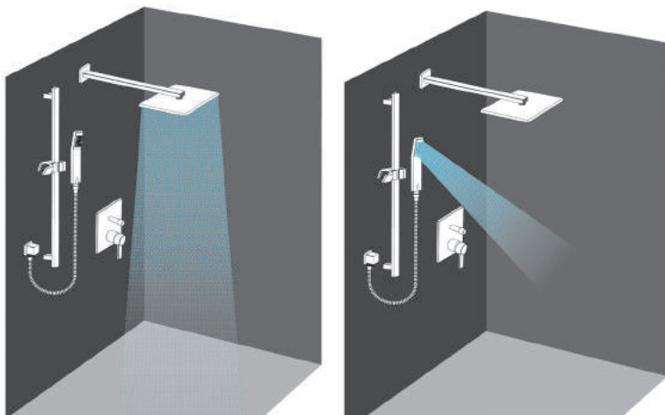
Ducha de empotrar con inversor. Rociador y teléfono. Concealed shower with diverter. Shower head and handset. Douche encastrée avec inverseur. Pomme de douche et douchette.
