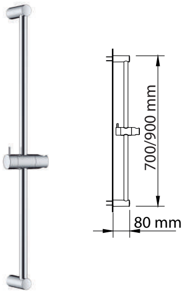
CITY BARRA DE DUCHA Sliding bar / Barre de douche
