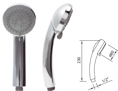
VIENNE | 3F | Ø80 mm DUCHA | Handset | Douchette
