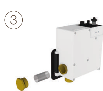
Limpieza de filtro Filter cleaning / Nettoyage du filtre
