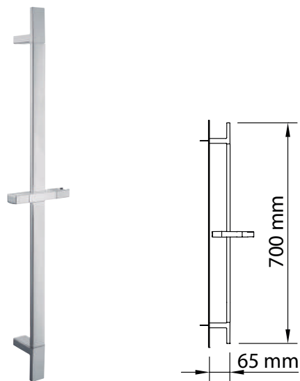
TREND 30x10x700 mm BARRA DE DUCHA Sliding bar Barre de douche
