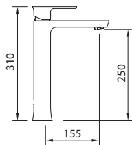
LAVABO 250 Tall basin mixer 250 | Mitigeur lavabo 250
