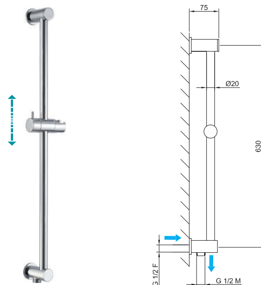
CITY - Ø20x715 mm BARRA DE DUCHA EMPOTRADA Concealed sliding bar Barre de douche encastré
