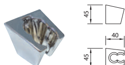
S12 SOPORTE FIJO Fix holder Support douchette fixe
