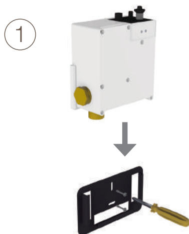
Sujeción caja pared Wall box fixing / Fixation de la boîte murale
