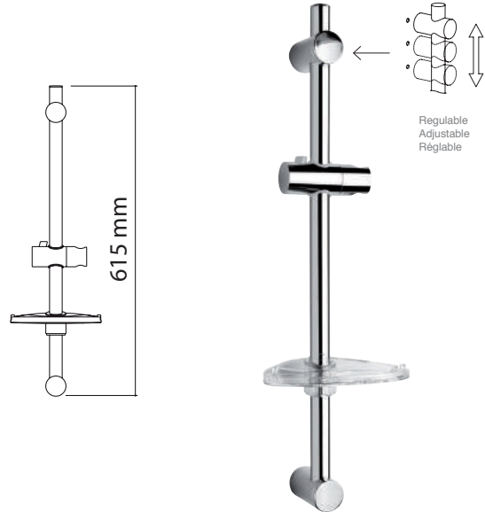
EIRE ø25x615 mm BARRA DE DUCHA Sliding bar / Barre de douche
